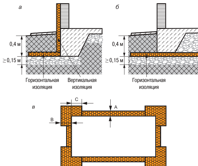
Рис. 2. Морозозащищенные фундаменты мелкого заложения: а – отапливаемых зданий; б – неотапливаемых зданий; в – параметры теплоизоляционного слоя
